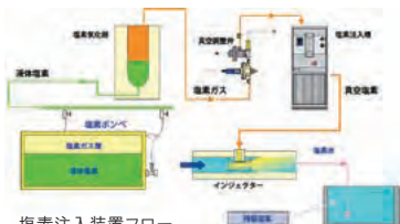
塩素注入装置フロー
